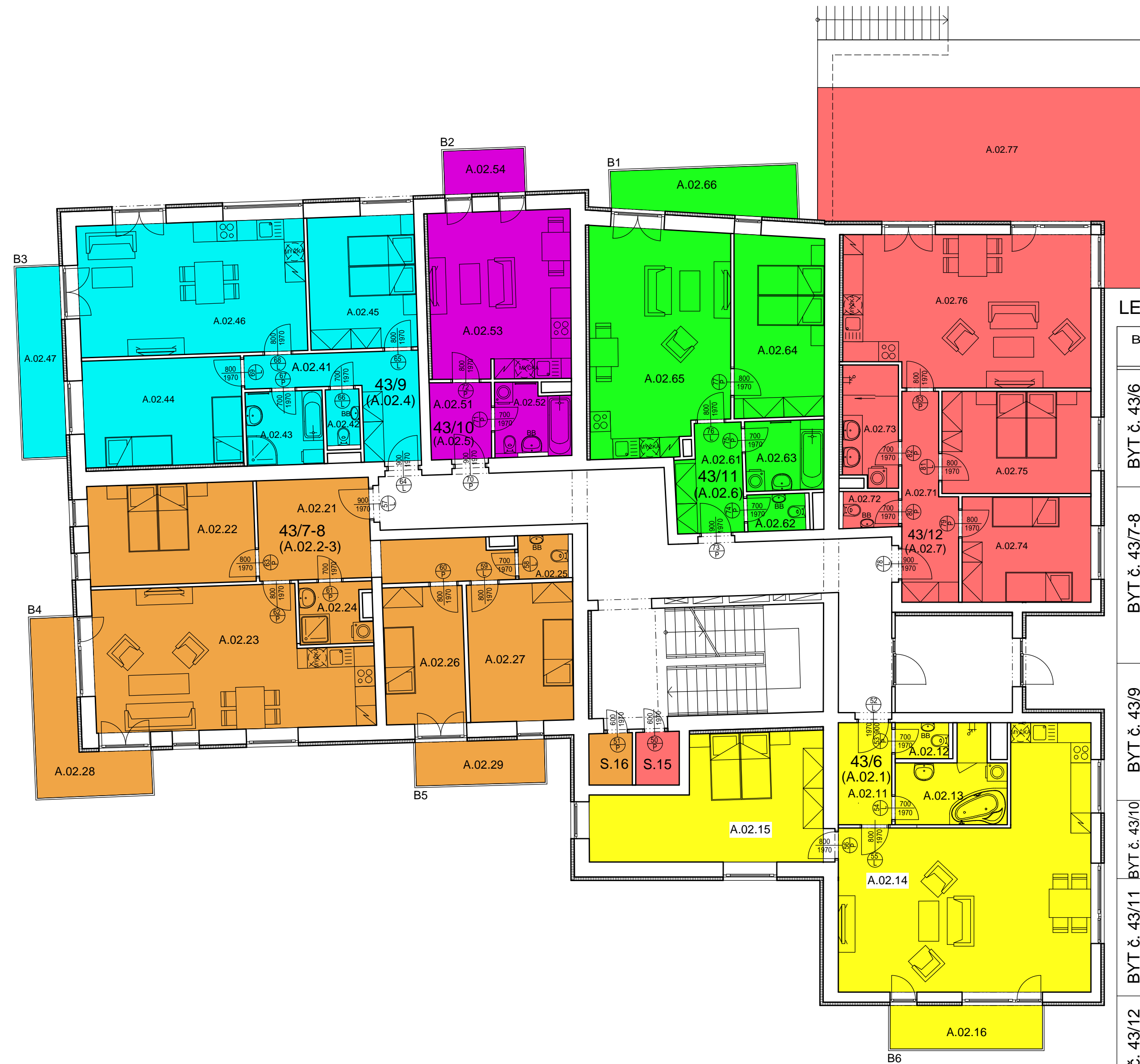
A - PŮDORYS 2.NP
